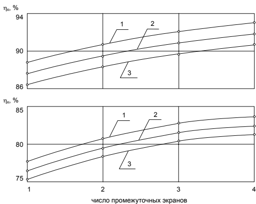
Рис. 3. Изменение КПД котла в зависимости от количества промежуточных экранов и температуры наружного воздуха: 1 - t_{нар} = +20 °С; 2 - t_{нар} = -10 °С; 3 - t_{нар} = -40 °С --- КВа-1,74 ГМ; — КВр-1,16 К
